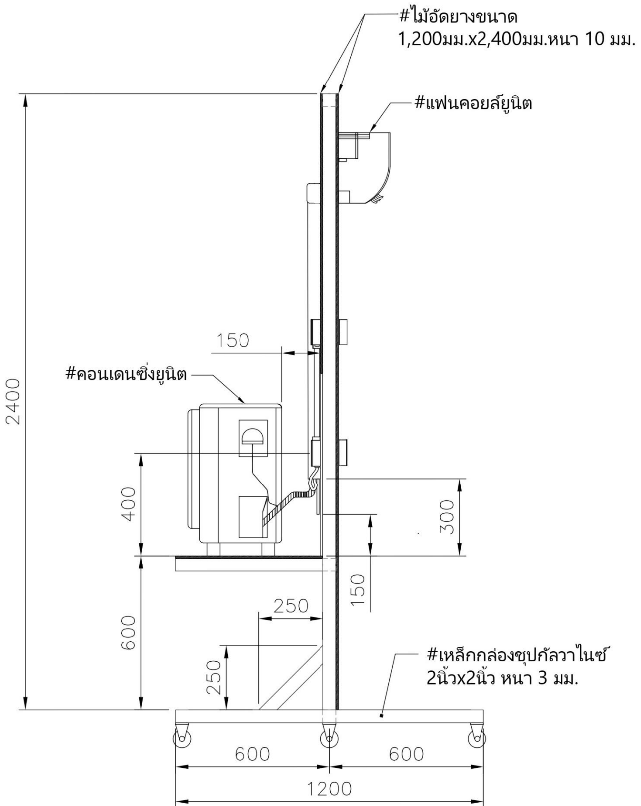
ภาพด้านข้าง (SIDE VIEW)
