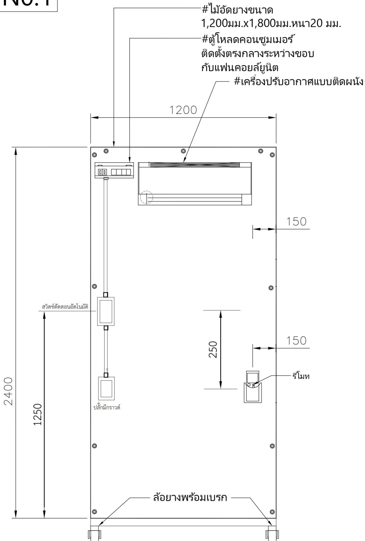
ภาพด้านหน้า (FRONT VIEW)
