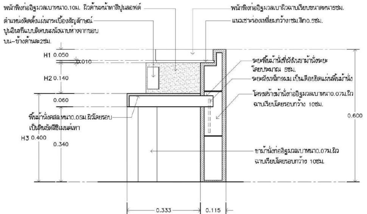
รูปตัดแนว A-A มาตราส่วน 1:10
